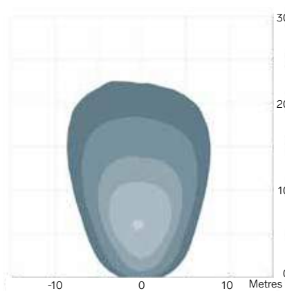
D10 / 2500 lm Medium 31-45° 3.0 m / -15° Symmetric
